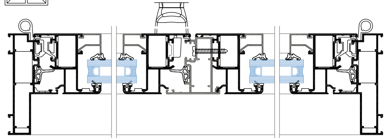
Ventana de abrir de 2 hojas
