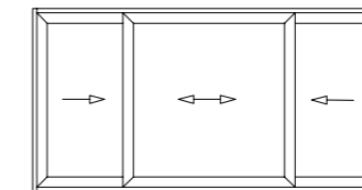
3 hojas en 2 guías
