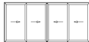
Corrediza 4 hojas en 2 guías
